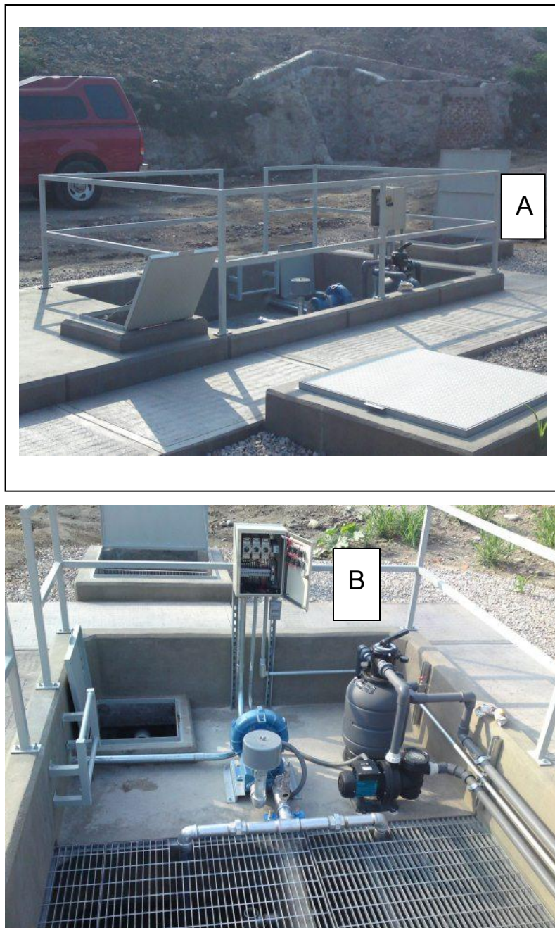
Figura 1.2 Fotografías de la PTAR Modelo BioNautilus: (A) vista lateral de la PTAR; (B) Biorreactores, red de aireación y soplador.
