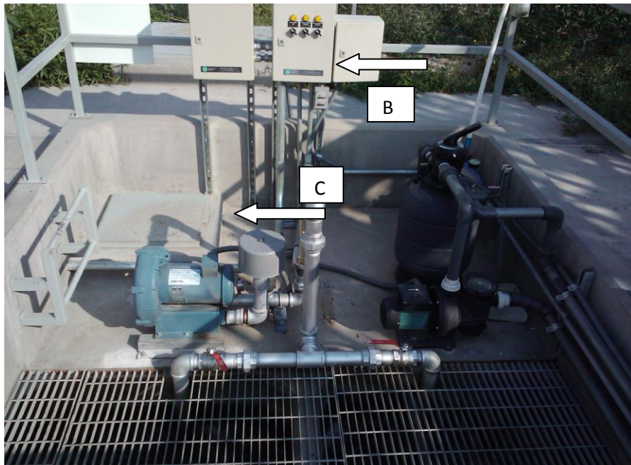
Figura 3.5 Foto de rotámetro(A), motovariador (B) y modificación a la red de aire (C)
